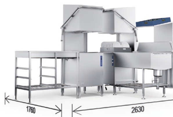
WD-6フード食器洗い機を備えたWD-PRM6プレリンス機
